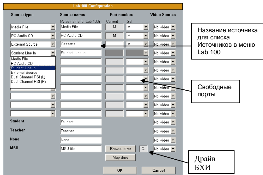
Окно конфигурирования Lab 100
